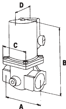
Rozměrový výkres VE4000A1 Série
