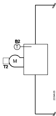
1° hořák
