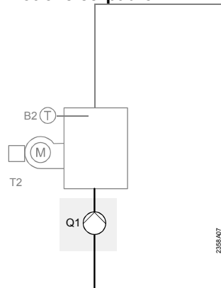
Kotlové čerpadlo
