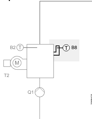
Spalinové čidlo
