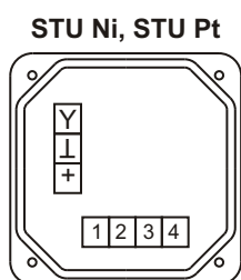
2-vodičové zapojení
