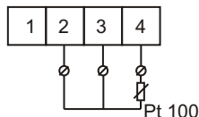
3-vodičové zapojení
