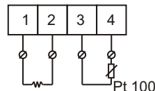
Zapojení s kompenzační smyčkou
