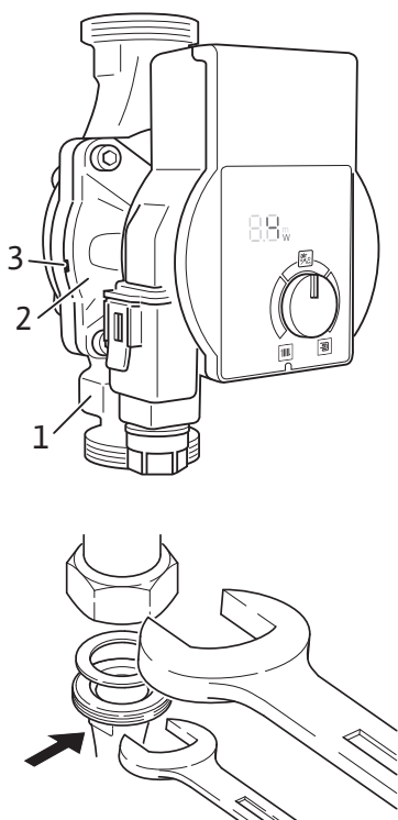
Fig. 4: Instalace čerpadla
